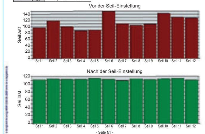
Abb. 6: Beispiel für einen Einstellreport des mobilen Seillastmesssystems WeightWatcher. In diesem Fall wurde ein Seilset von 12 Seilen eingestellt. Die max. Abweichung der Seile zueinander konnte von 17% auf 1% verbessert und somit frühzeitiger Verschleiß verhindert werden.
