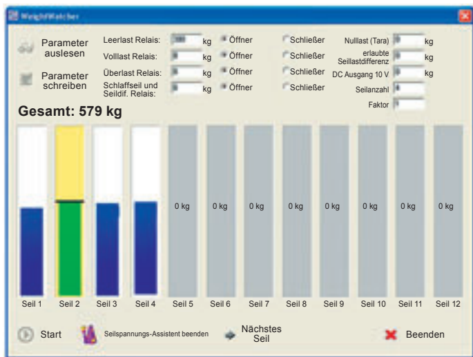
Abb. 4: ... sobald der Benutzer die vorgegebene Seilspannung eingestellt hat, wird dies visuell (grüner Balken) bestätigt und der Benutzer zum nächsten Seil und dessen Sollwert geführt. Sobald der Benutzer beim letzten Seil des Seilsets angekommen ist, ist die Seileinstellung abgeschlossen, ohne dass eines der Seile mehr als einmal eingestellt werden musste.
