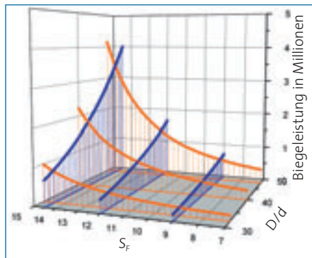
Abb. 1: Auswirkungen des Seildurchmessers ( S_r ) und des Verhältnisses von Treibscheibendurchmesser zu Seildurchmesser ( D/d ) auf die Biegeleistung 1)
