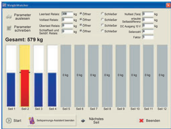
Abb. 3: Die Einstell-Software des stationären Lastmessgerätes AE12 gibt einen Seilspannungswert (schwarze Grenzlinie am roten Balken) vor, der vom Benutzer einzustellen ist ...
